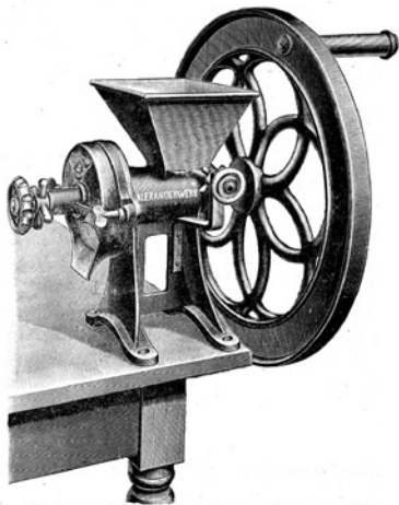
Młynek ręczny (srótkak do mielenia zboża a szczególnie pszenicy, gryki i t. p. Wydaje w godzinie do 15 kg. mielniwa – (cena 15 mk.).
